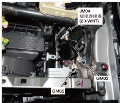
121. 仪表板右侧
