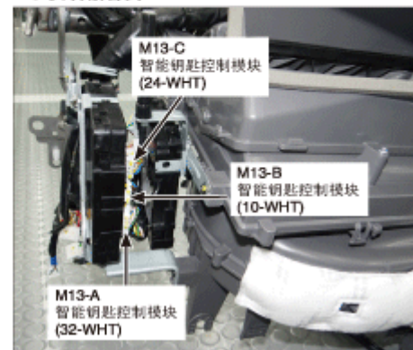
123. 仪表板右侧
