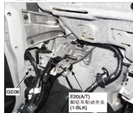
126. 防火板左侧
